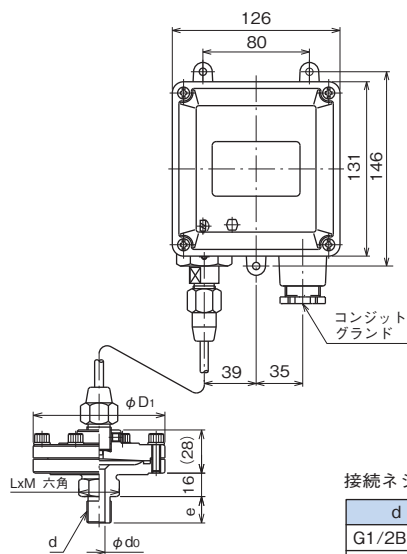
CQ30 圧カスイッチ
