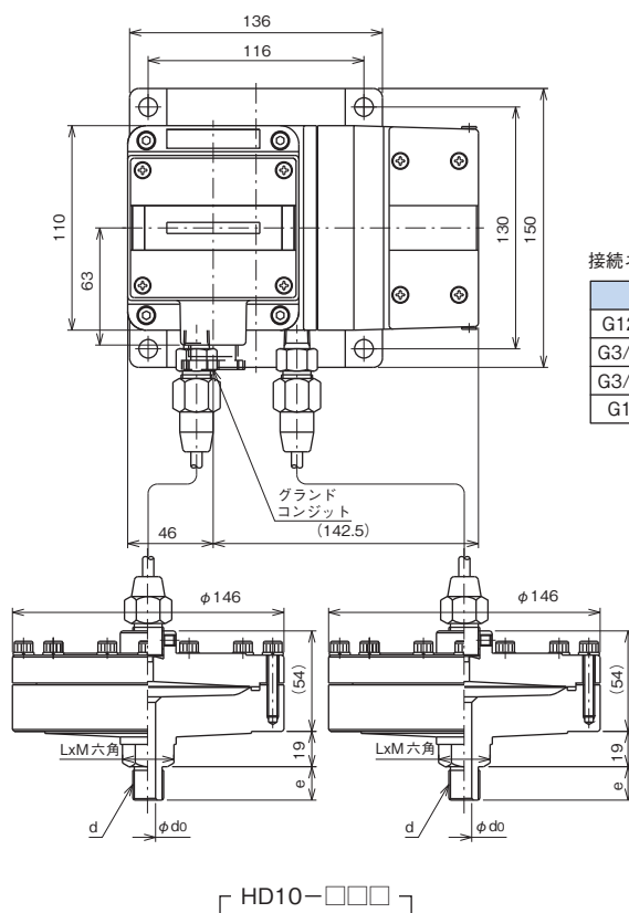
CL71 差圧スイッチ
