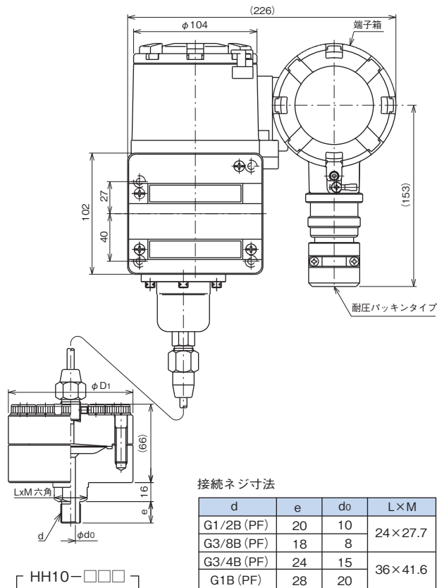
CD75 耐圧防爆形圧カスイッチ
