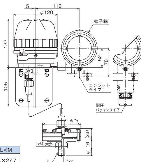
CD30 耐圧防爆形圧カスイッチ
