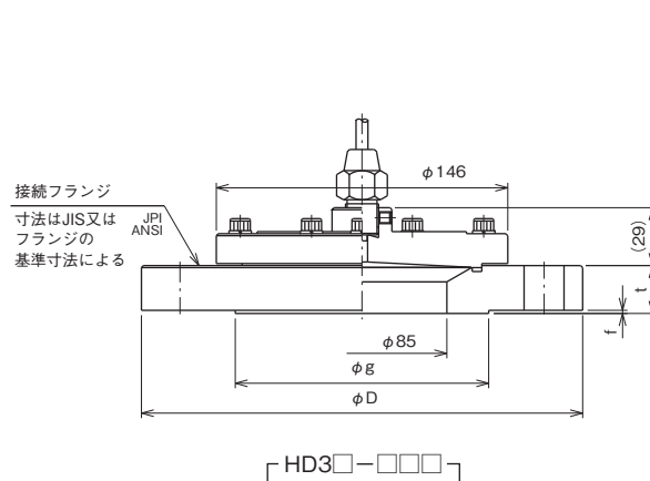
300形・フランジ
