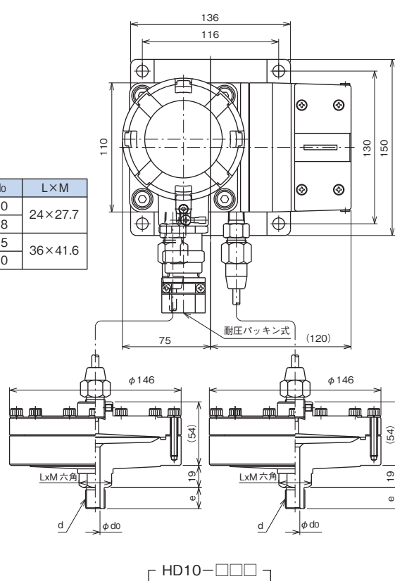
CD71 耐圧防爆形差圧カスイッチ
