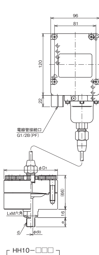
CB33 圧カスイッチ
