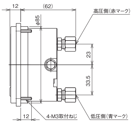
「DG70-261」 外径φ6銅管用継手
