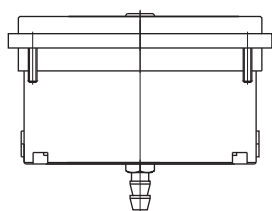
「DG70-291」 外径φ7タケノコ継手
