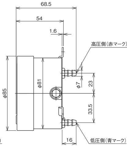
〔DG70-491〕 外径φ7タケノコ継手
