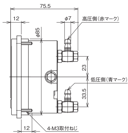
「DG70-211」 外径φ7タケノコ回転継手
