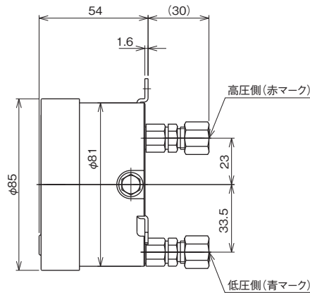
〔DG70-461〕 外径φ6銅管用継手
