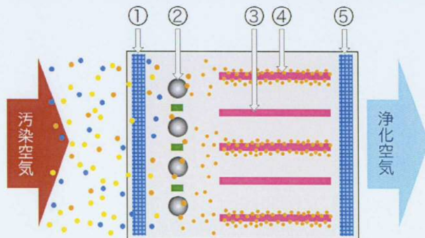
集塵機内部
